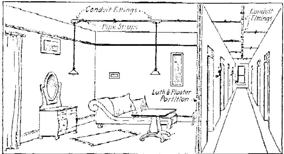
An exposed conduit
